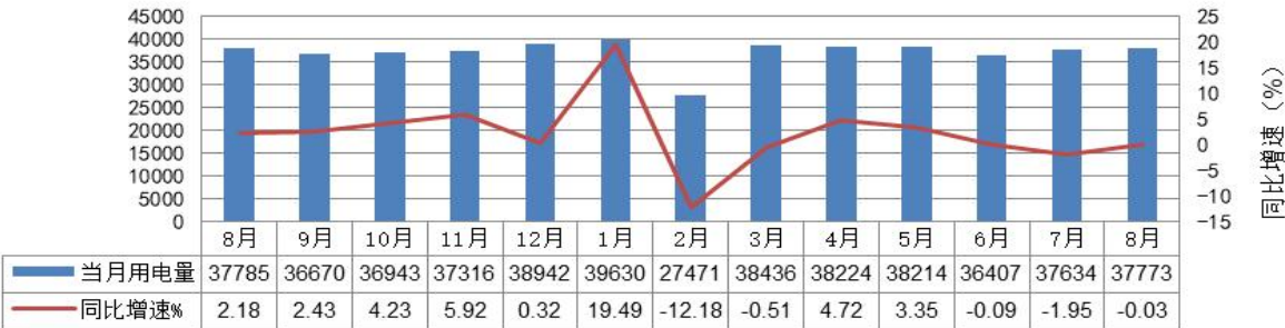
用电量走势图
